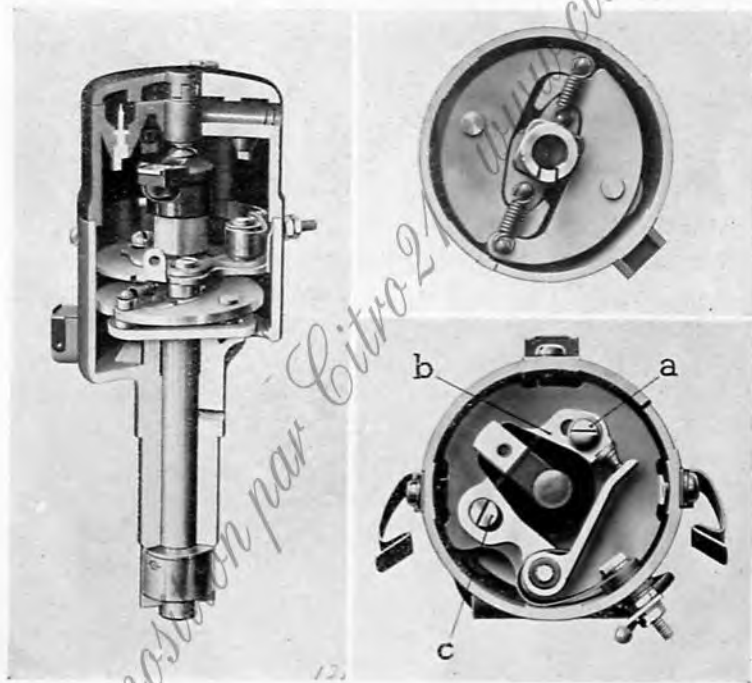
VUE EN COUPE DE L'ALLUMEUR
