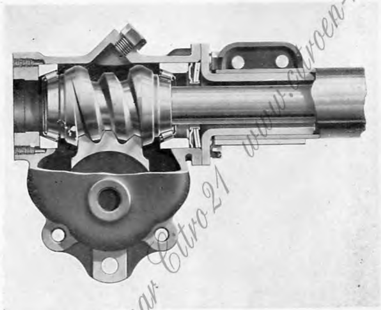
VUE EN COUPE DU BOITIER DE DIRECTION
