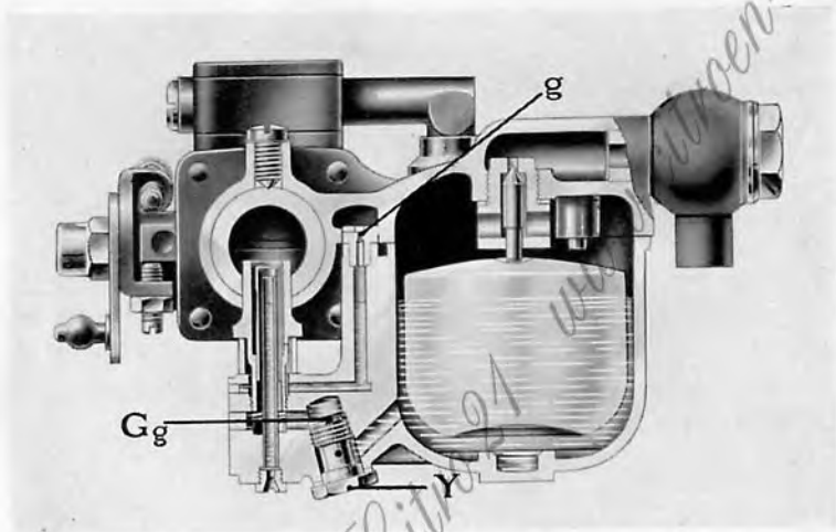
COUPE DU CARBURATEUR
